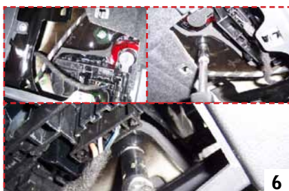
Bild 6 Innenteil der Leuchte von der Heckklappe demontieren, dazu die 3 Verschraubungen lösen, Mutter auf Gewindestück M8. Remove the interior piece proceeding to with the 3 screws, screw sockets onto threaded part.
