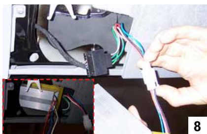
Bild 8 Neues Innenteil anschließen und mitgeliefertes Steuermodul in die Serviceöffnung einsetzen und mit den beiden unteren Befestigungsschrauben verschrauben und verbinden Sie das Steuermodul am freien Stecker. New inner part and use the included control module connected to the service port and fix it with the two lower mounting screws. Connect the control module on the free plug.
