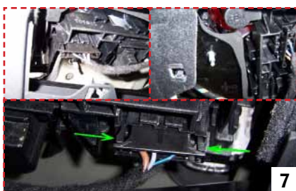
Bild 7 Stecker vom Innenteil lösen, dazu seitlich die zwei Rastnasen drücken und Stecker abziehen. Release the connector from the inner part, press side locking pins and remove the connector.
